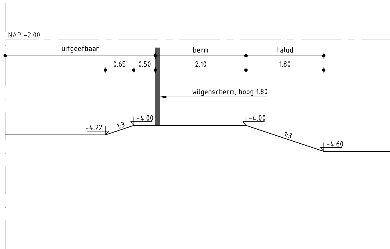
principe detail erfafscheiding schiphol parkeren schaal 1:50
